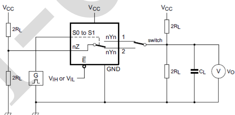
a. Test circuit
